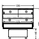
Areor® ST 1253 G (Vorderansicht)
