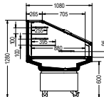
Areor® ST 1253 G (Seitenansicht)
