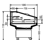
Areor® SD 1253 G (Seitenansicht)
