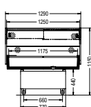
Areor® SD 1253 G (Vorderansicht)
